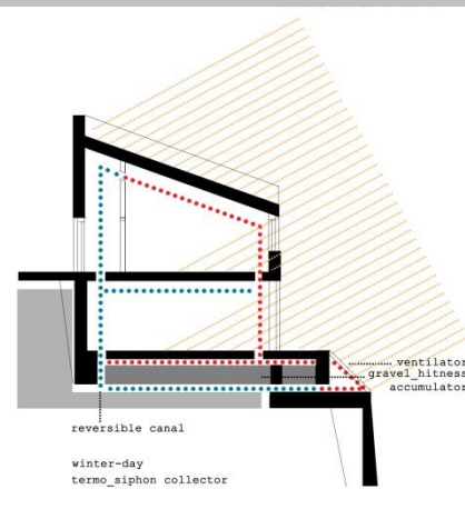
Термосифонски колектор
